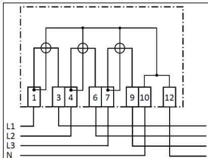
Abb. 2: Schaltung 4000 (Eintarif)
