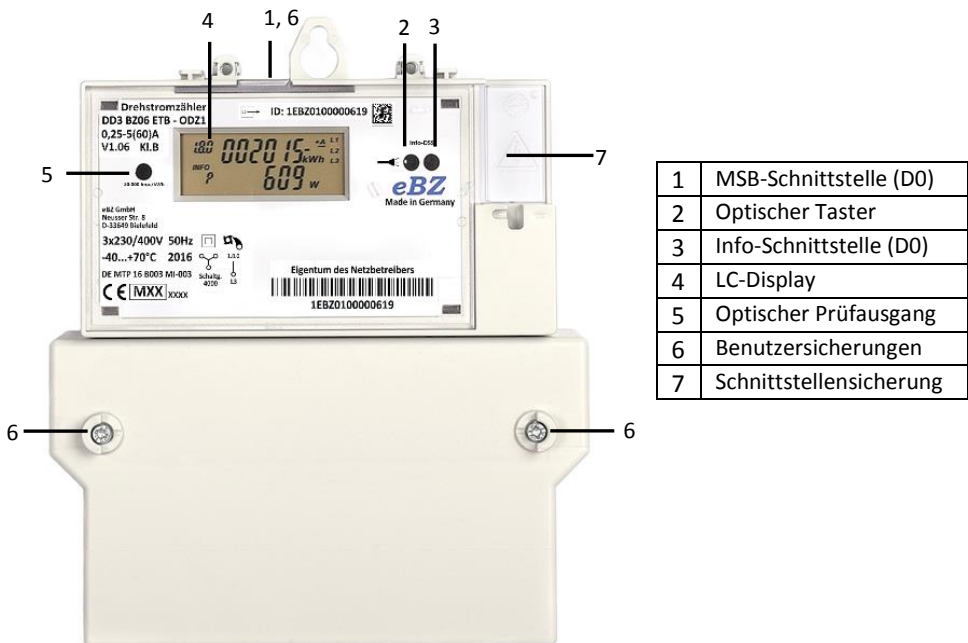
Abb. 1: Merkmale des Zählers DD3
