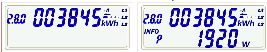
Abb. 9: Anzeige Lieferzähler ohne (links) und mit (rechts) Leistungsanzeige
