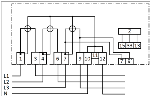
Abb. 3: Schaltung 4102 (Doppeltarif)
