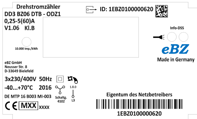
Abb. 4: Leistungsschild des DD3 (Beispiel)
