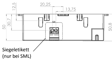
DD3 mit Zusatzklemmen
